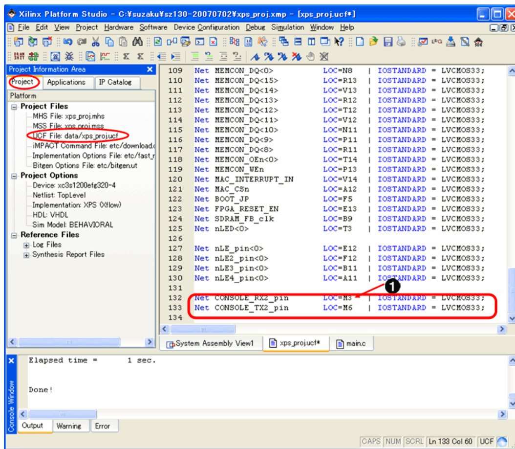
図 10.83. UART(xps_proj.ucf)
