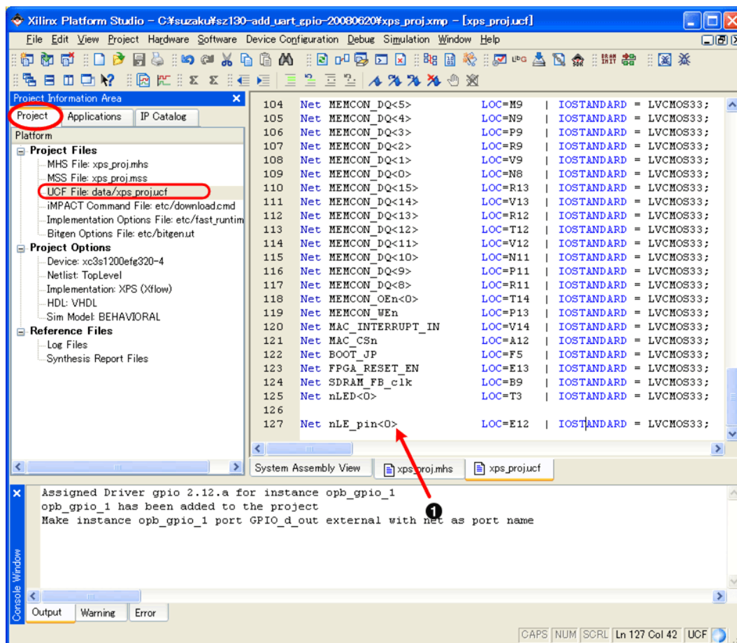
図 10.53. GPIO(xps_proj.ucf)
