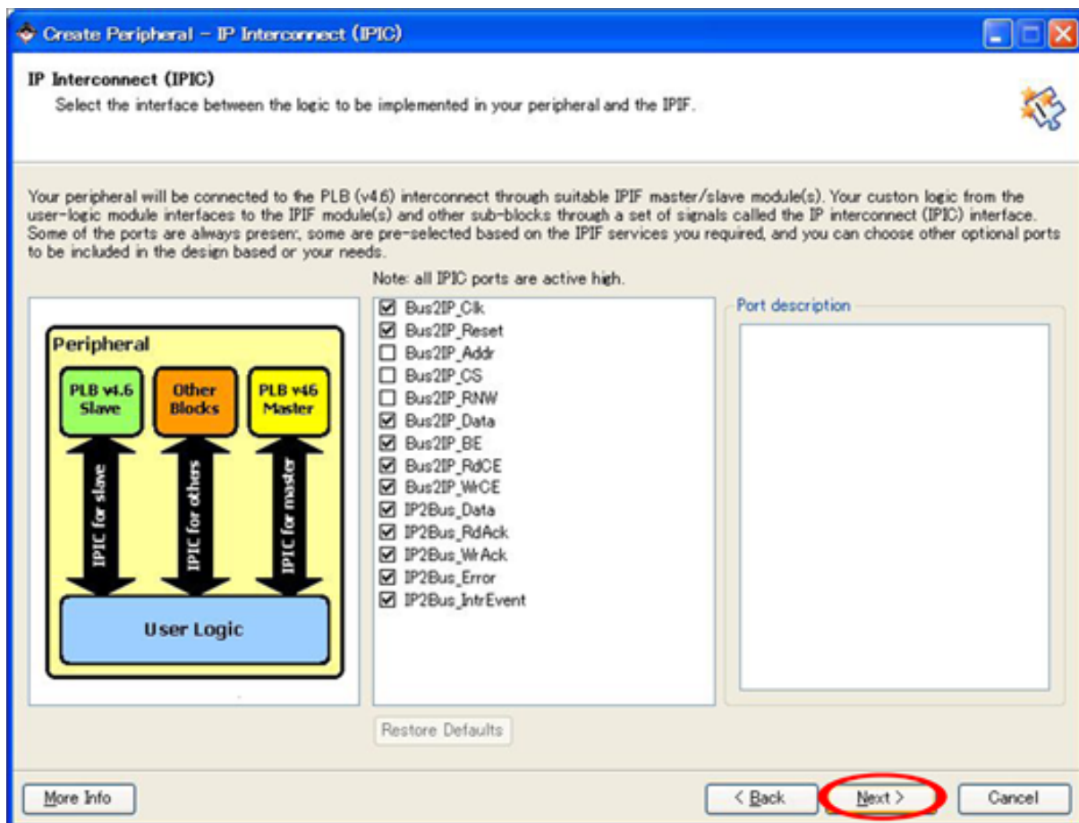
図 11.31. IPIC 設定
