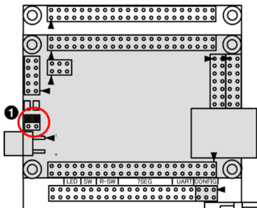
図 5.3. ブートローダモード ジャンプの設定
