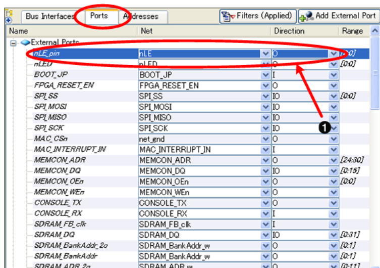
図 10.52. 信号名変更
