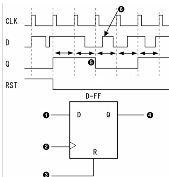
図 8.7. D-FF の動作
