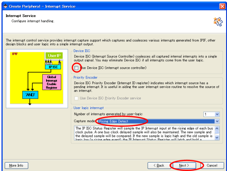
図 11.10. Interrupt 設定
