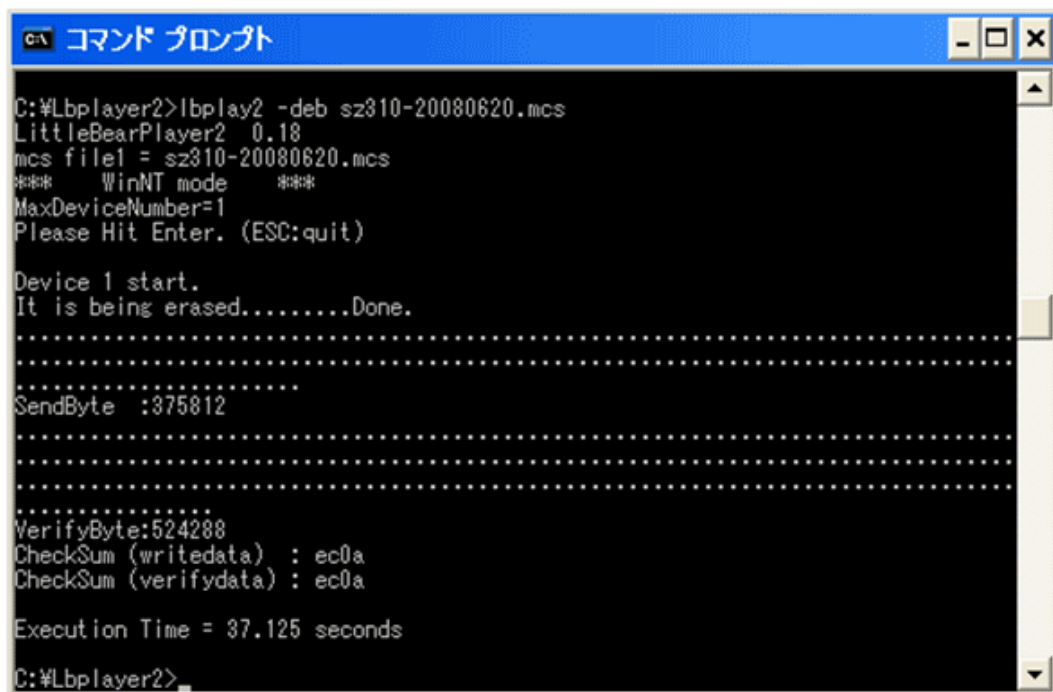
図 6.24. LBPlay2 実行
