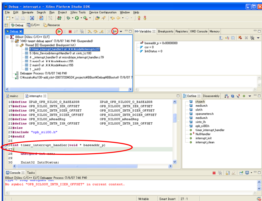
図 12.29. timer_interrupt_handler で Break
