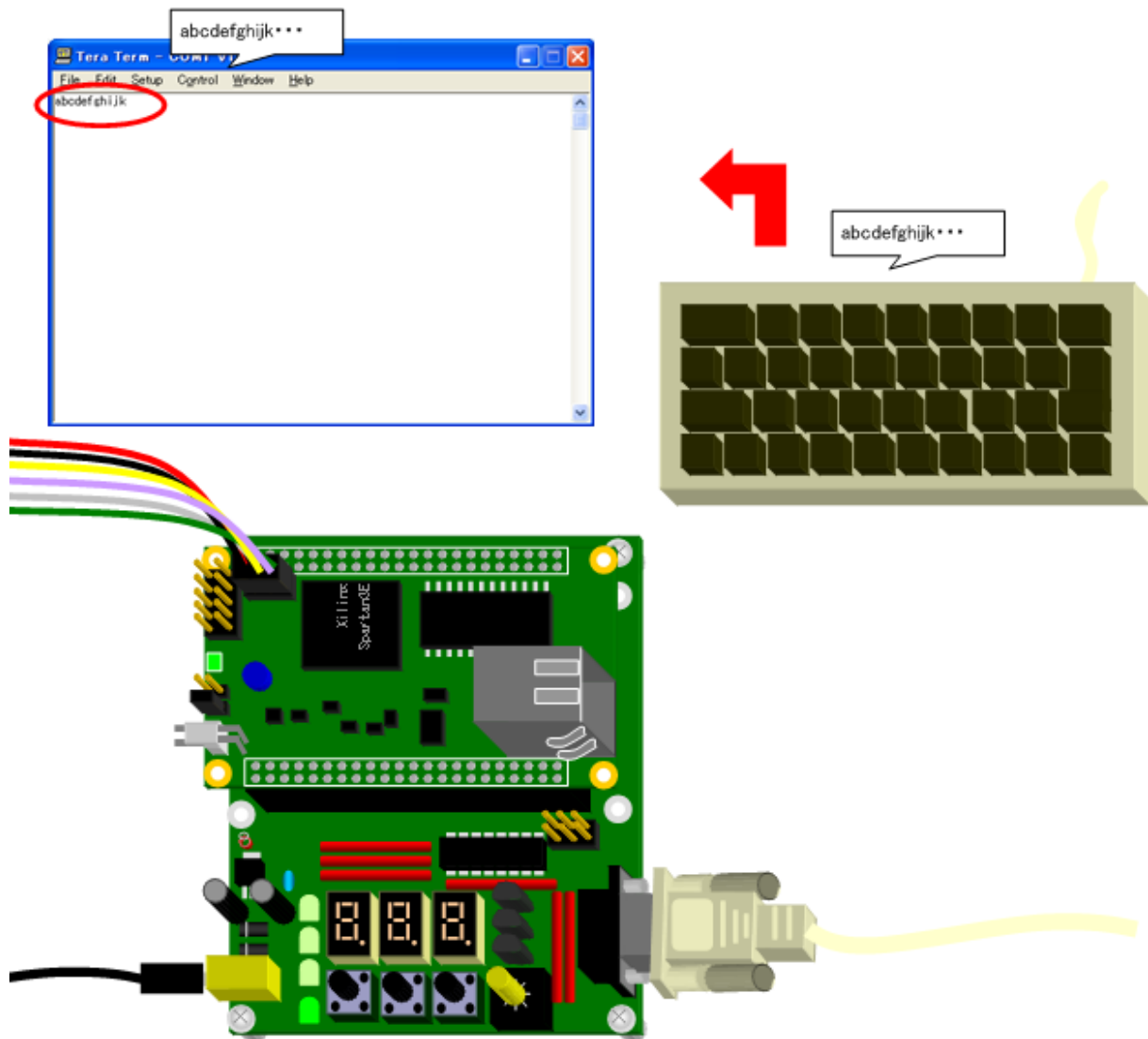
図 10.88. シリアル通信 動作確認
