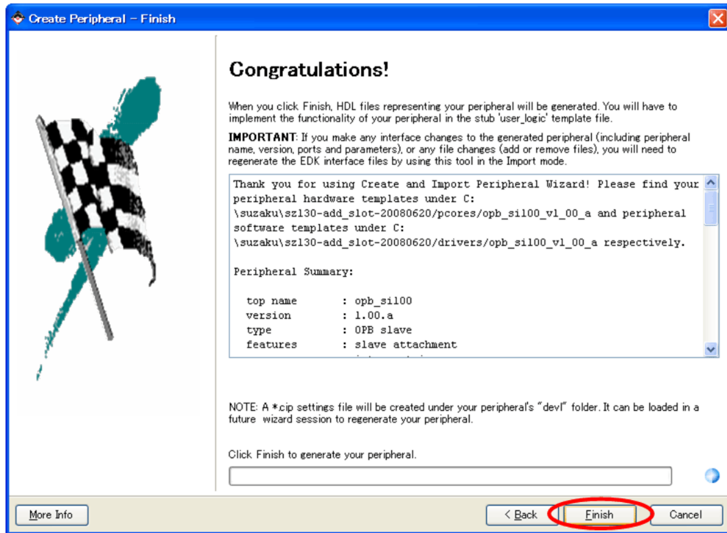
図 11.15. 終了
