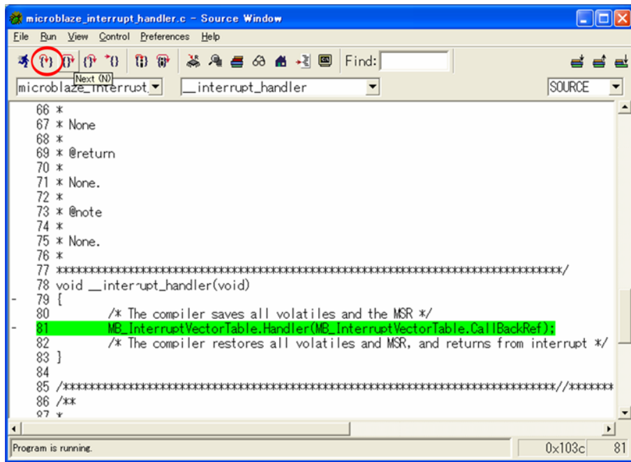
図 11.92. _interrupt_handler() で Break
