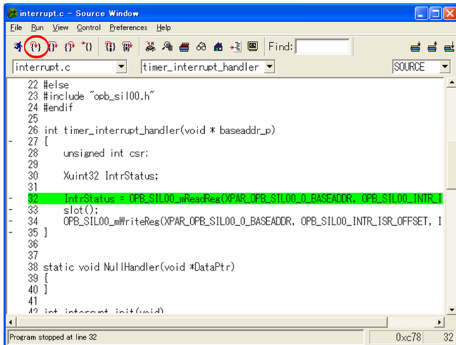
図 11.94. timer_interrupt_handler( )で Break
