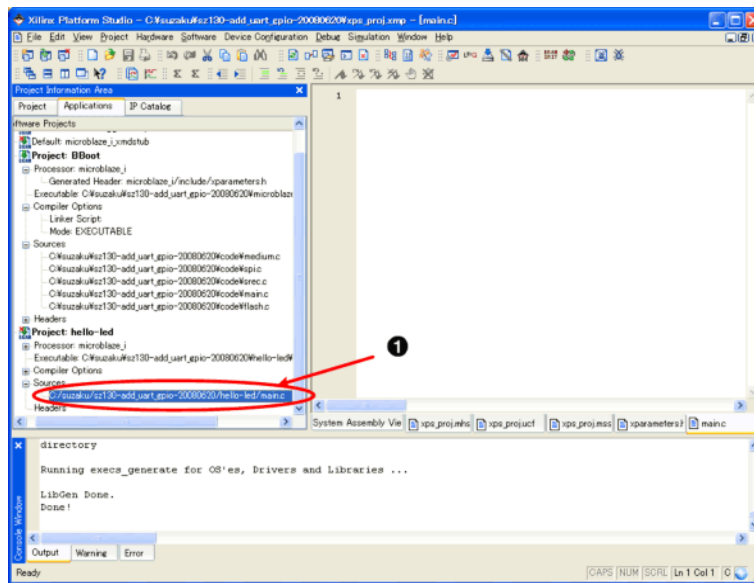
図 10.62. main.c を開く
