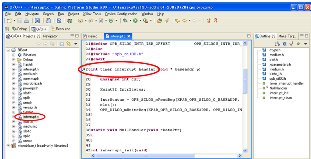
図 12.23. BreakPoint 設定
