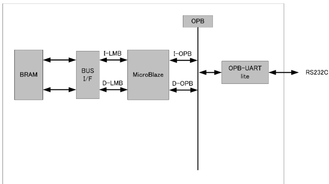
図 10.2. Hello SUZAKU プロジェクト(MicroBlaze)
