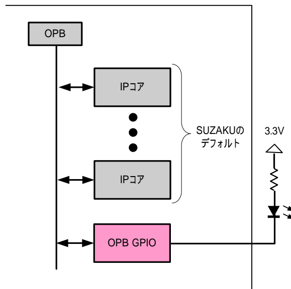
図 10-35 GPIO を追加して LED を点灯
