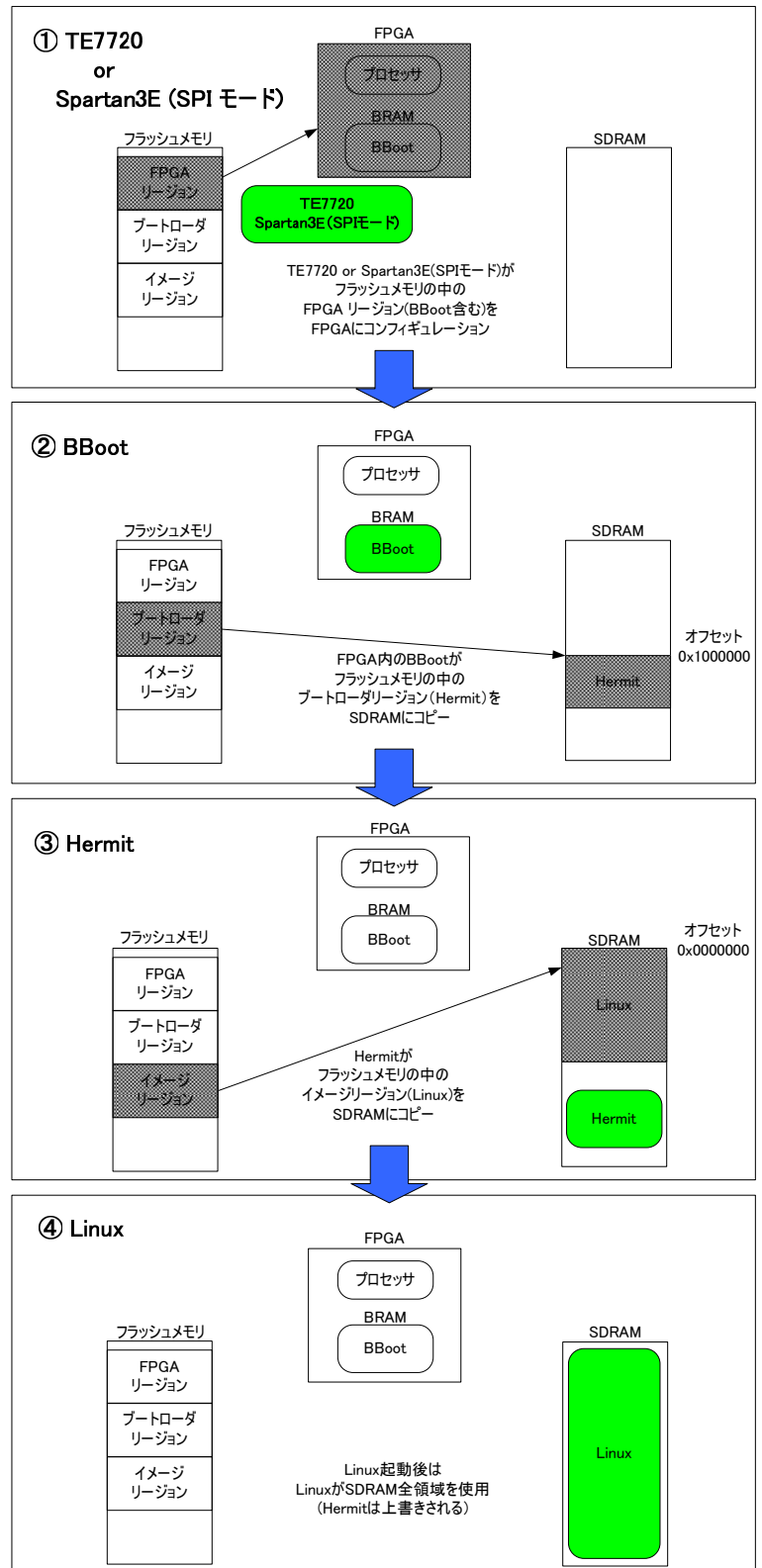
図 5-11 2 段階ブート
