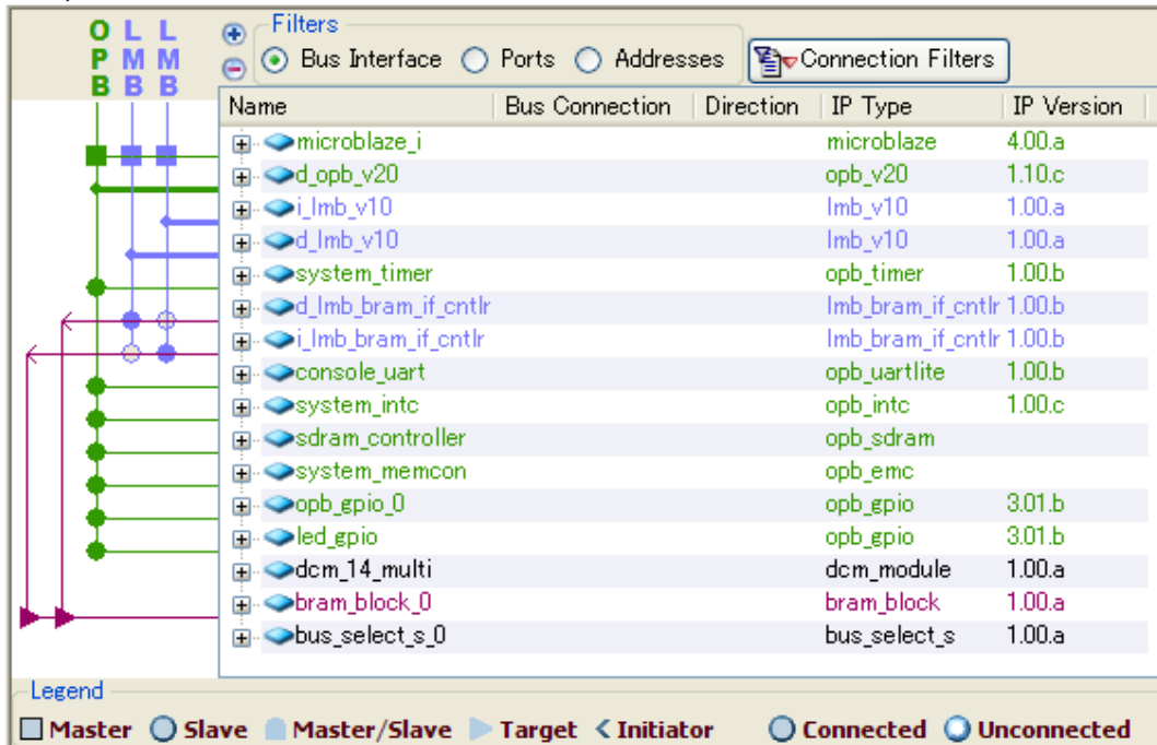
図 10-28 SZ010, SZ030 のデフォルト(EDK)
