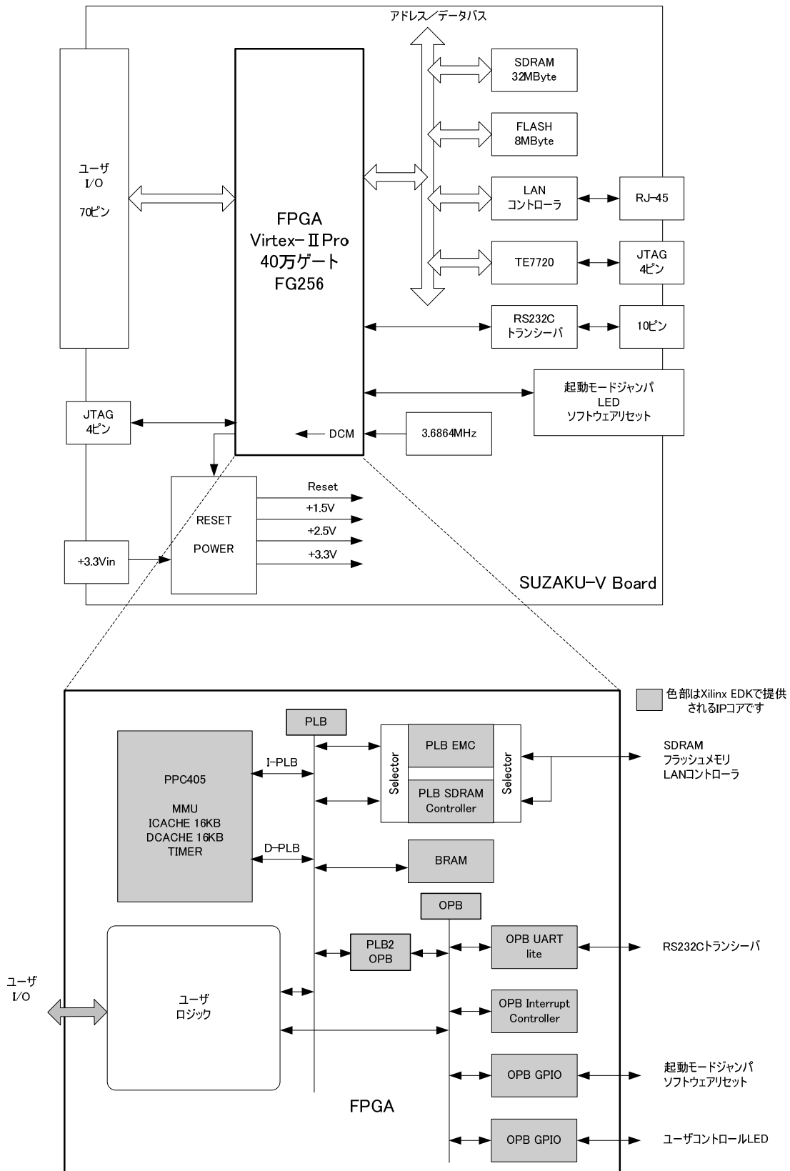
図 1-9 SZ310 の全体ブロック図
