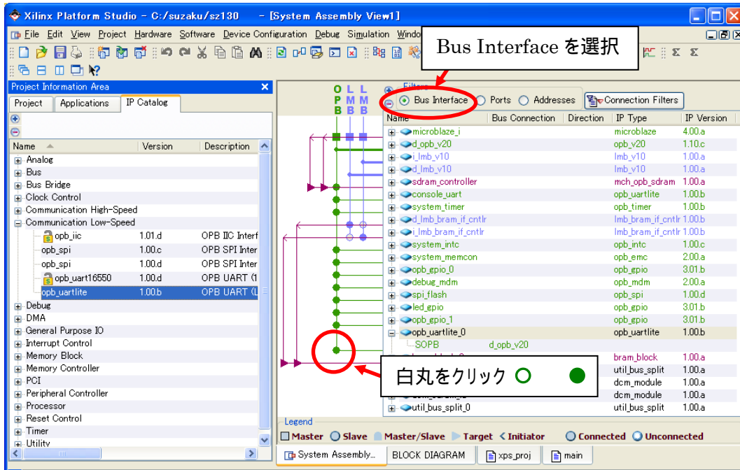
図 10-71 OPB バスに接続
