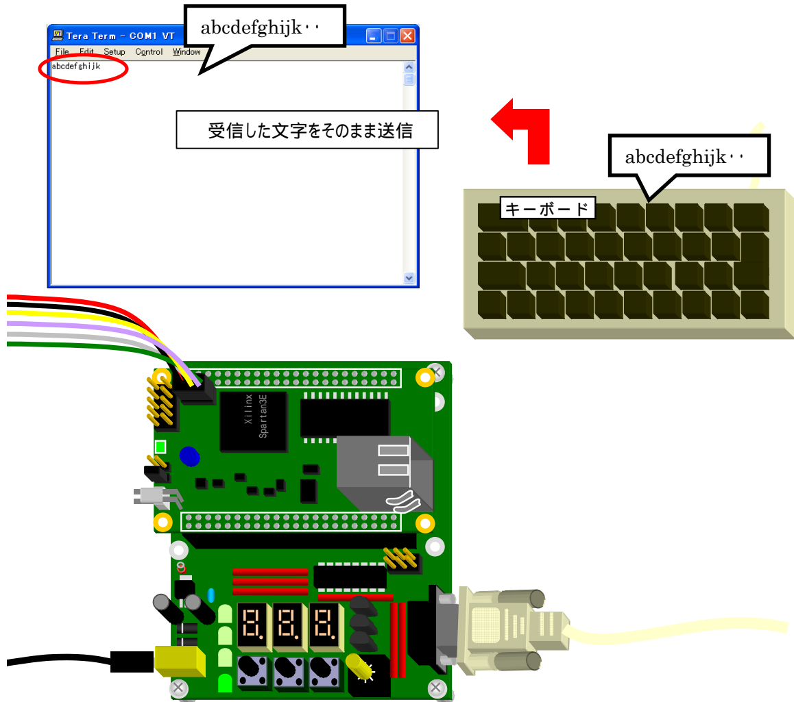
図 10-83 シリアル通信 動作確認
