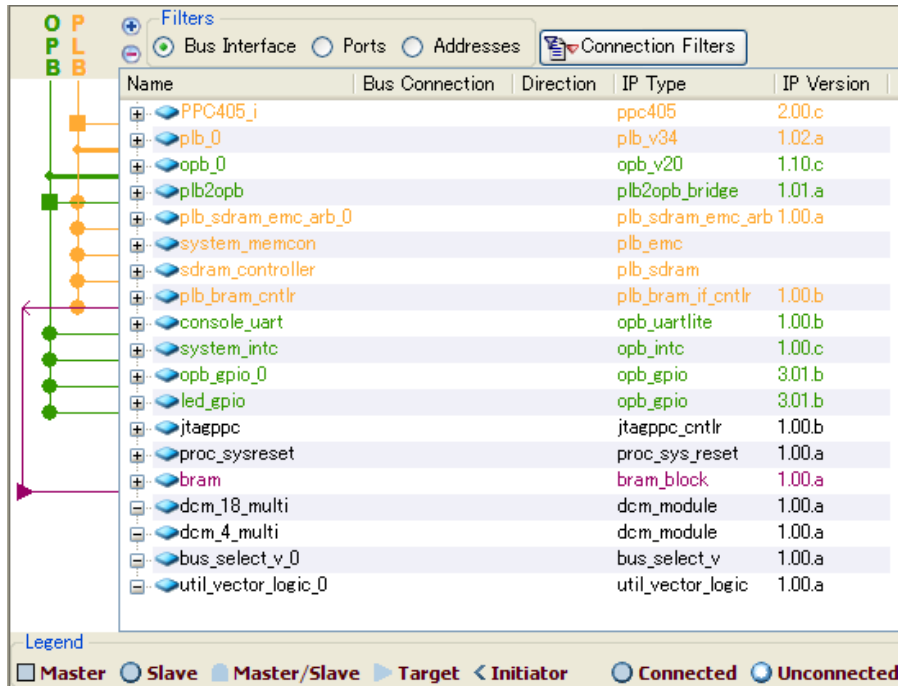
図 10-32 SZ310 のデフォルト(EDK)
