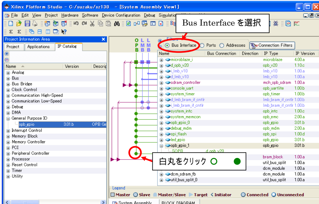
図 10-37 OPB バスに接続
