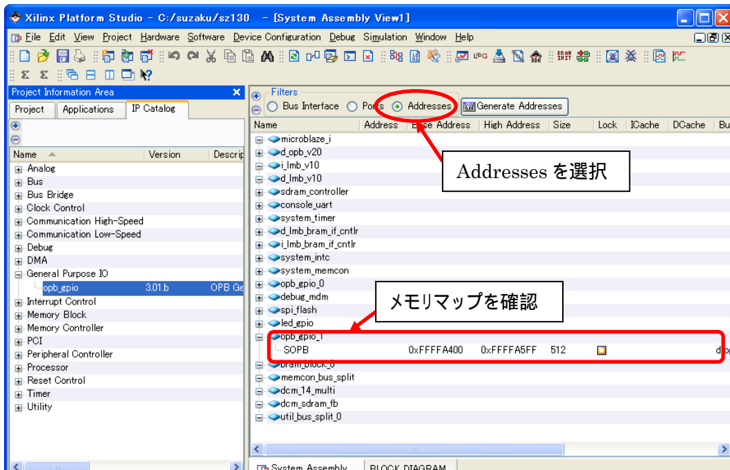
図 10-43 メモリマップ確認
