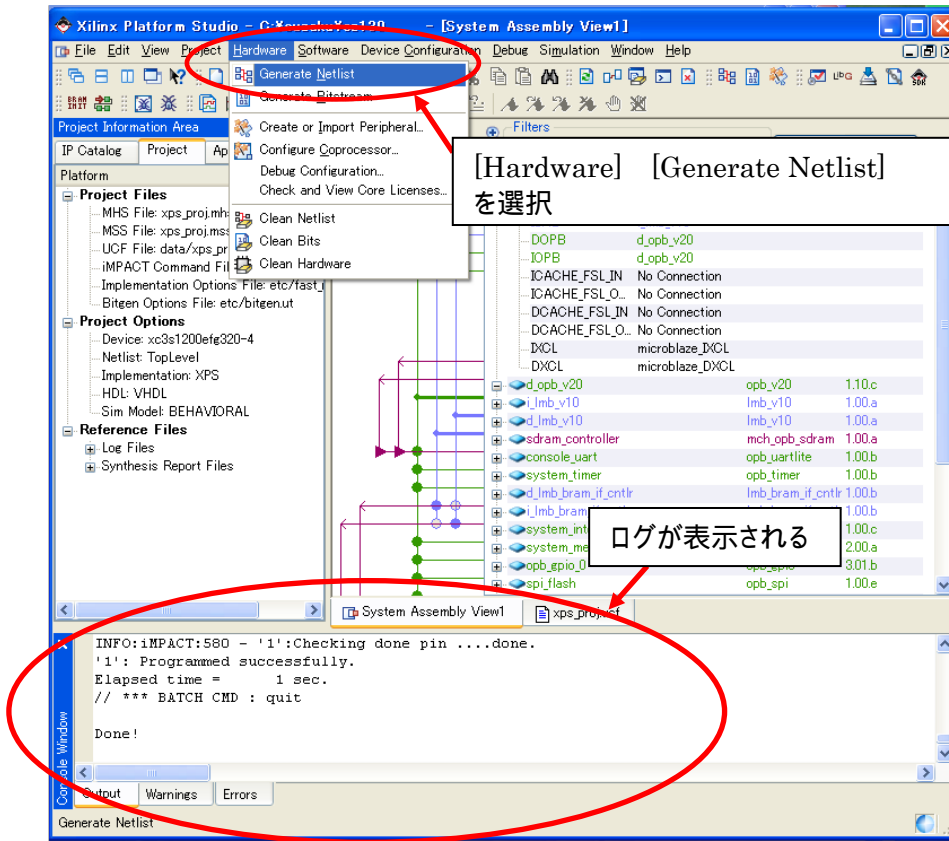
図 10-48 ネットリスト作成
