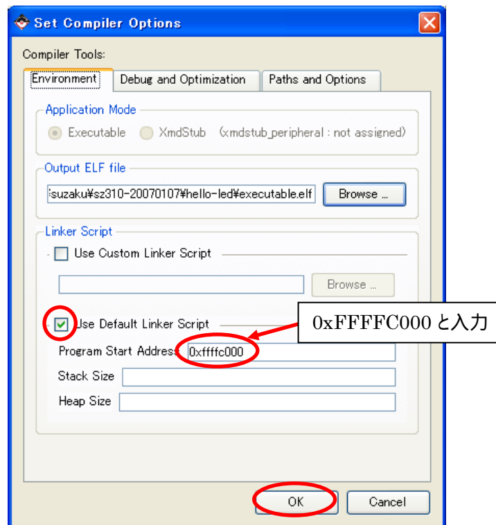
図 10-61 スタートアドレス設定
