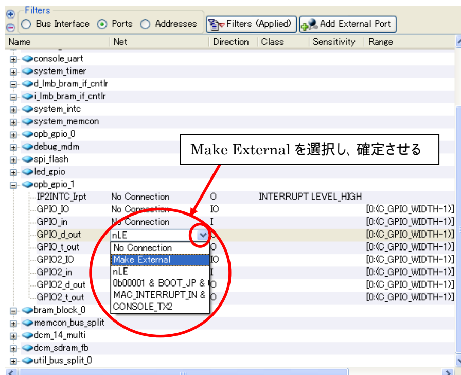
図 10-45 外部信号にする
