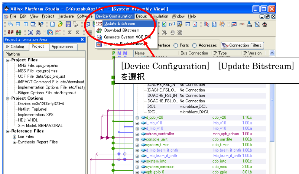
図 10-63 bit ファイル作成
