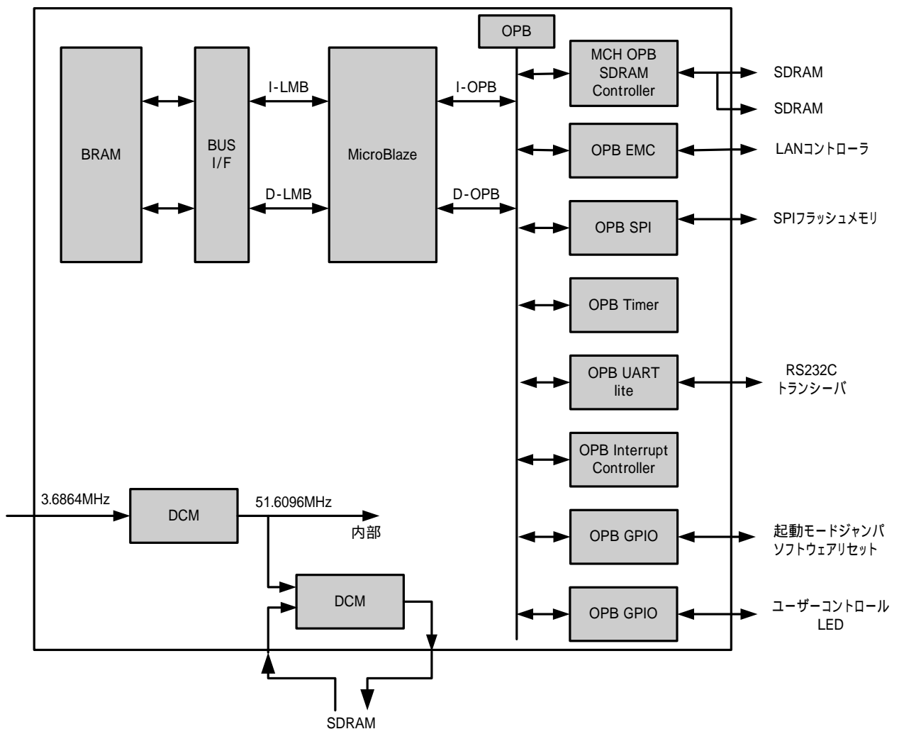
図 10-31 SZ130 デフォルトのブロック図
