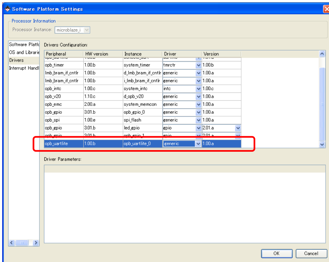
図 10-79 UART Driver 設定
