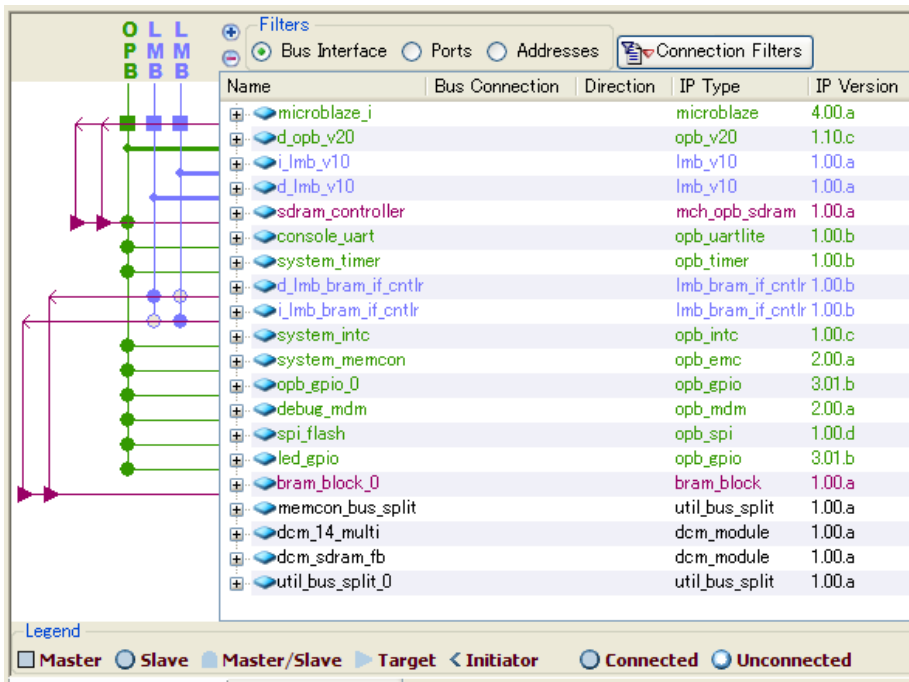
図 10-30 SZ130 のデフォルト(EDK)
