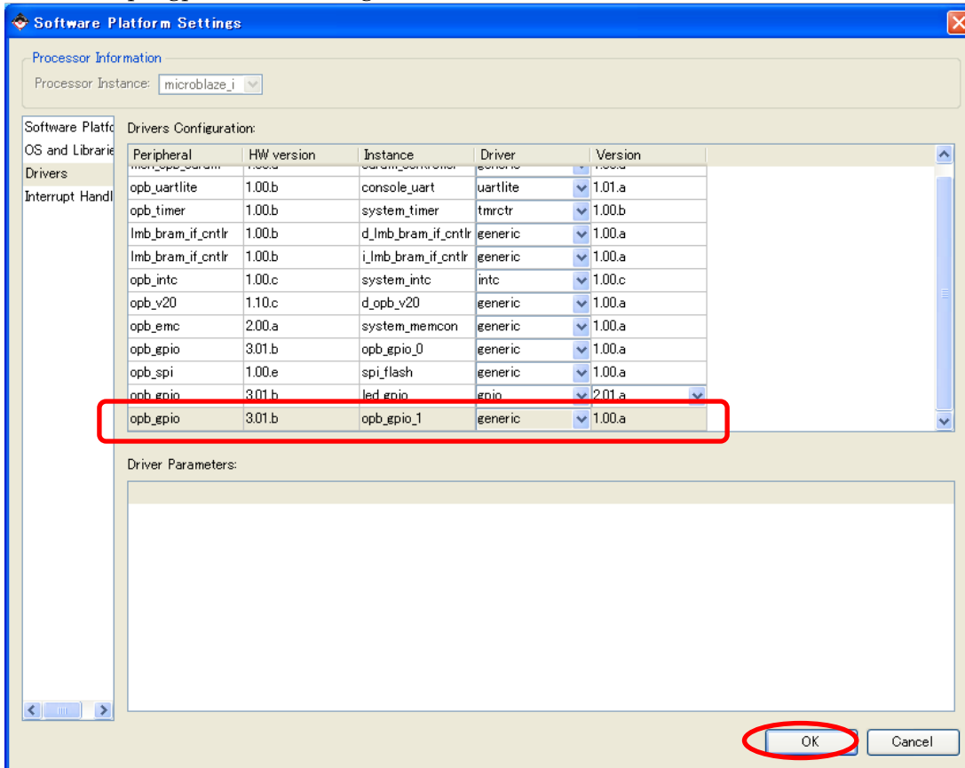
図 10-50 GPIO Driver 設定
