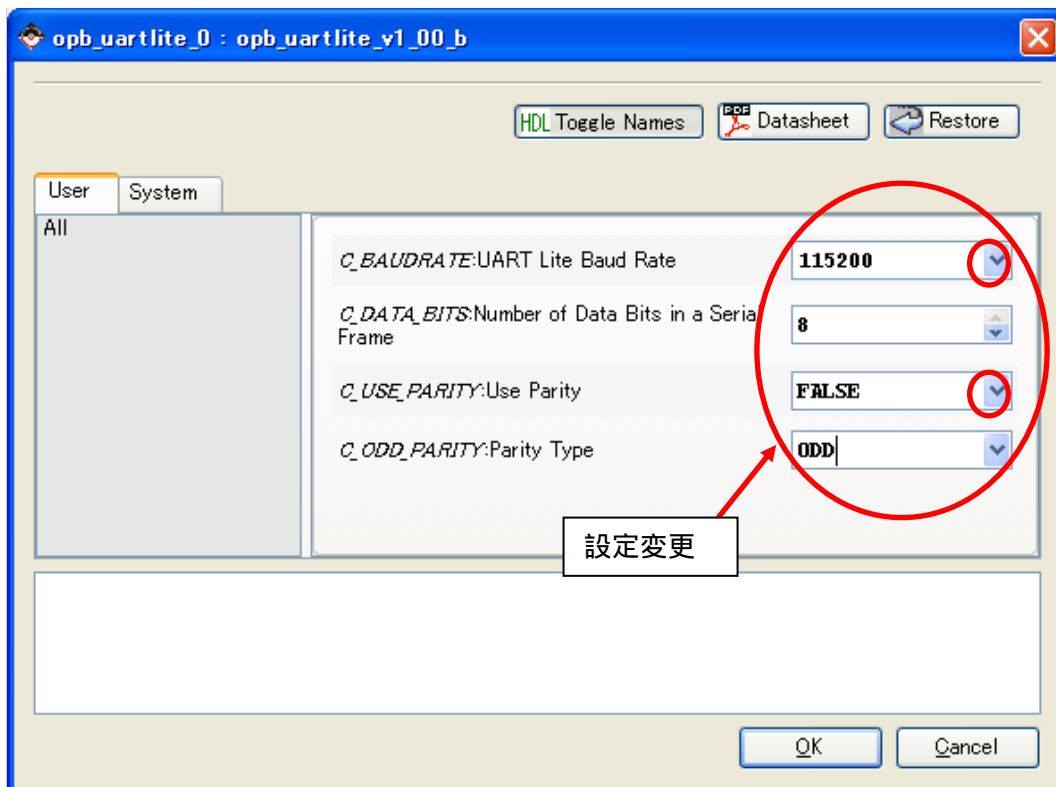
図 10-73 UART 設定変更
