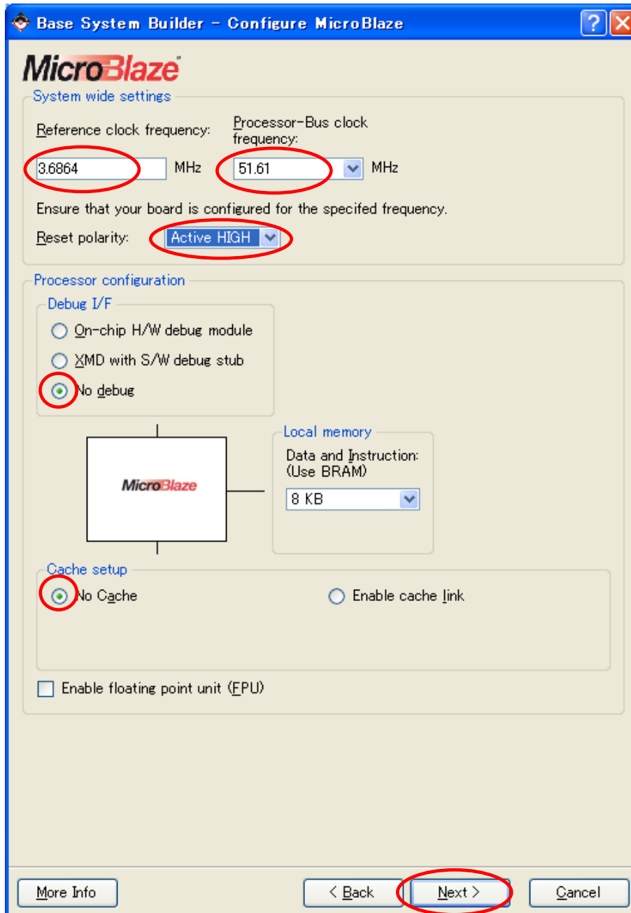
図 10-8 MicroBlaze の設定
