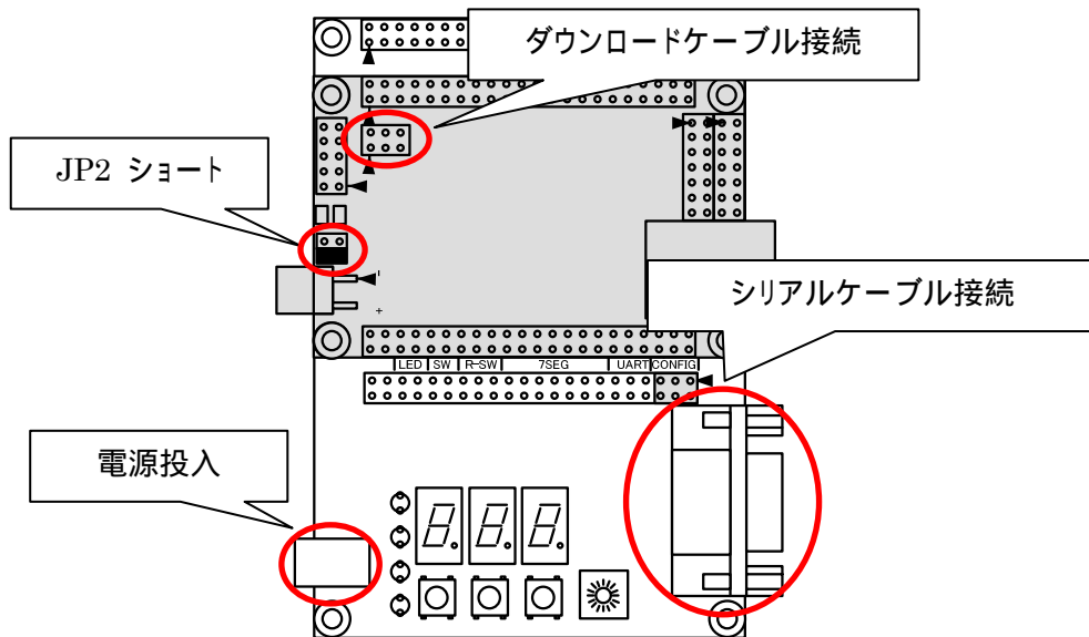
図 10-82 ジャンパの設定等
