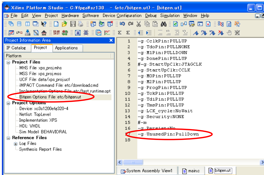
図 10-67 Bitgen のオプション設定
