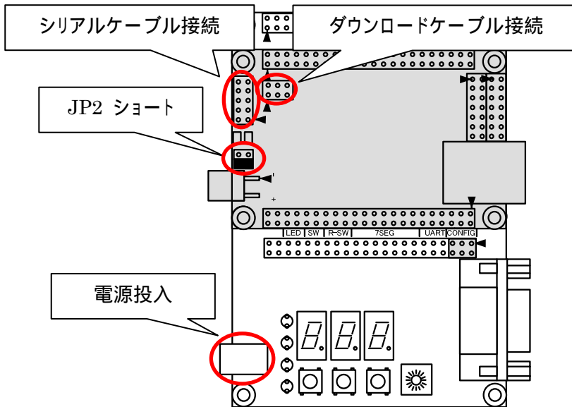
図 10-24 ジャンパの設定等
