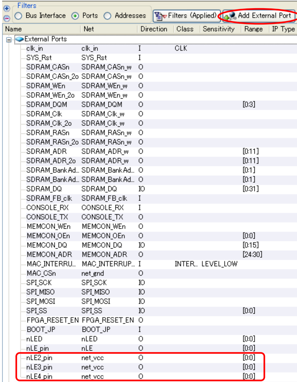
図 10-68 EDK での空きピンの処理
