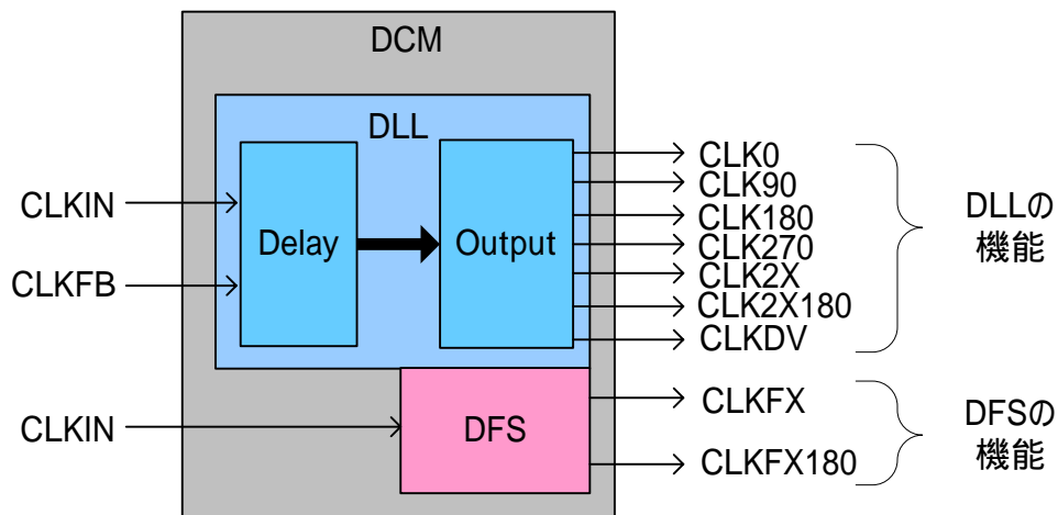
図 10-18 DCM の一部
