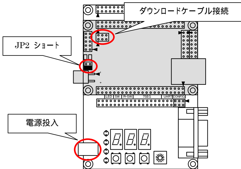
図 10-64 ジャンパの設定等
