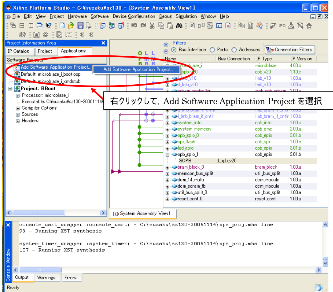
図 10-52 アプリケーション作成
