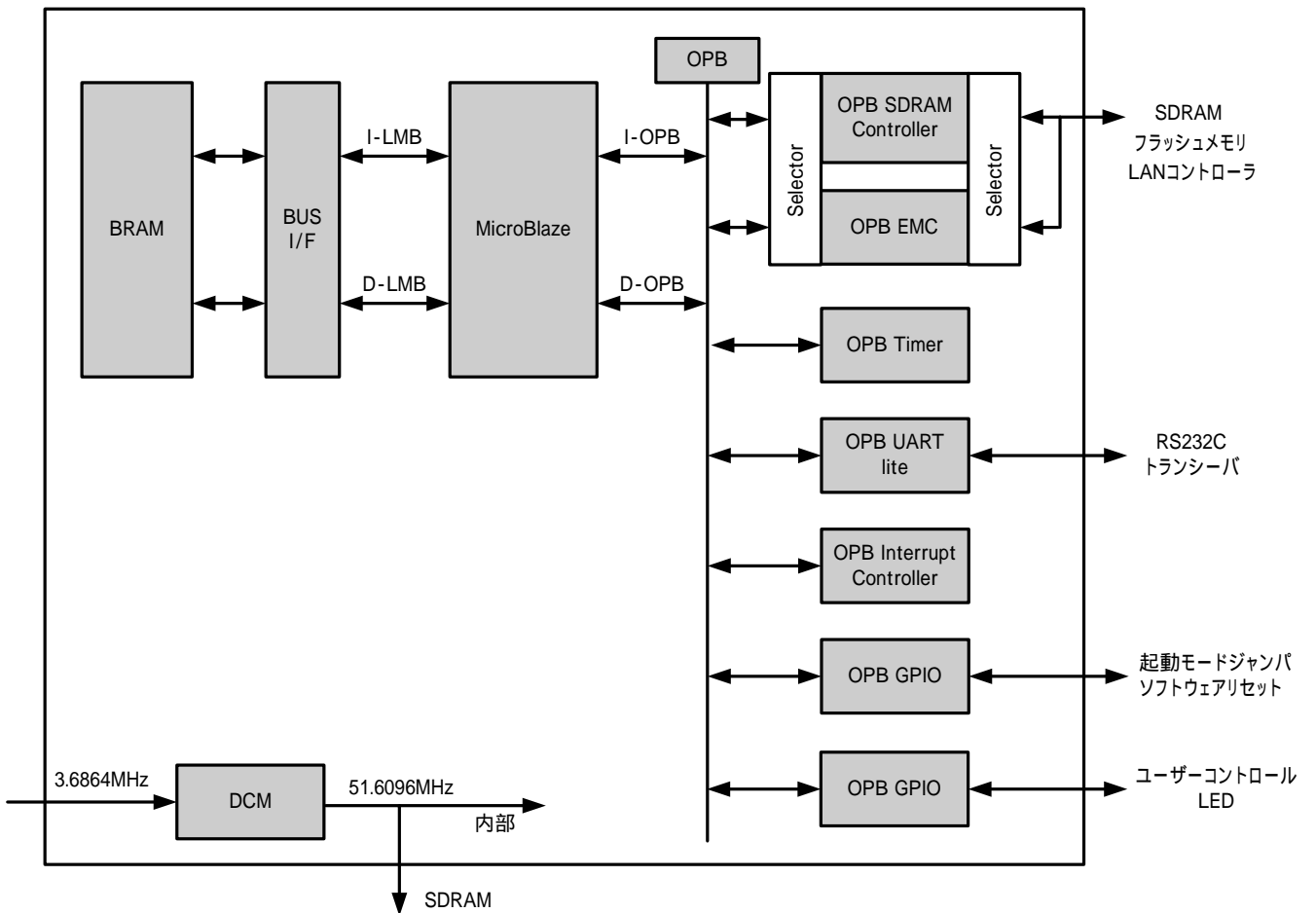
図 10-29 SZ010, SZ030 デフォルトのブロック図
