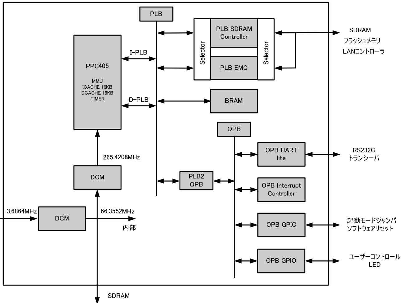
図 10-33 SZ310 デフォルトのブロック図
