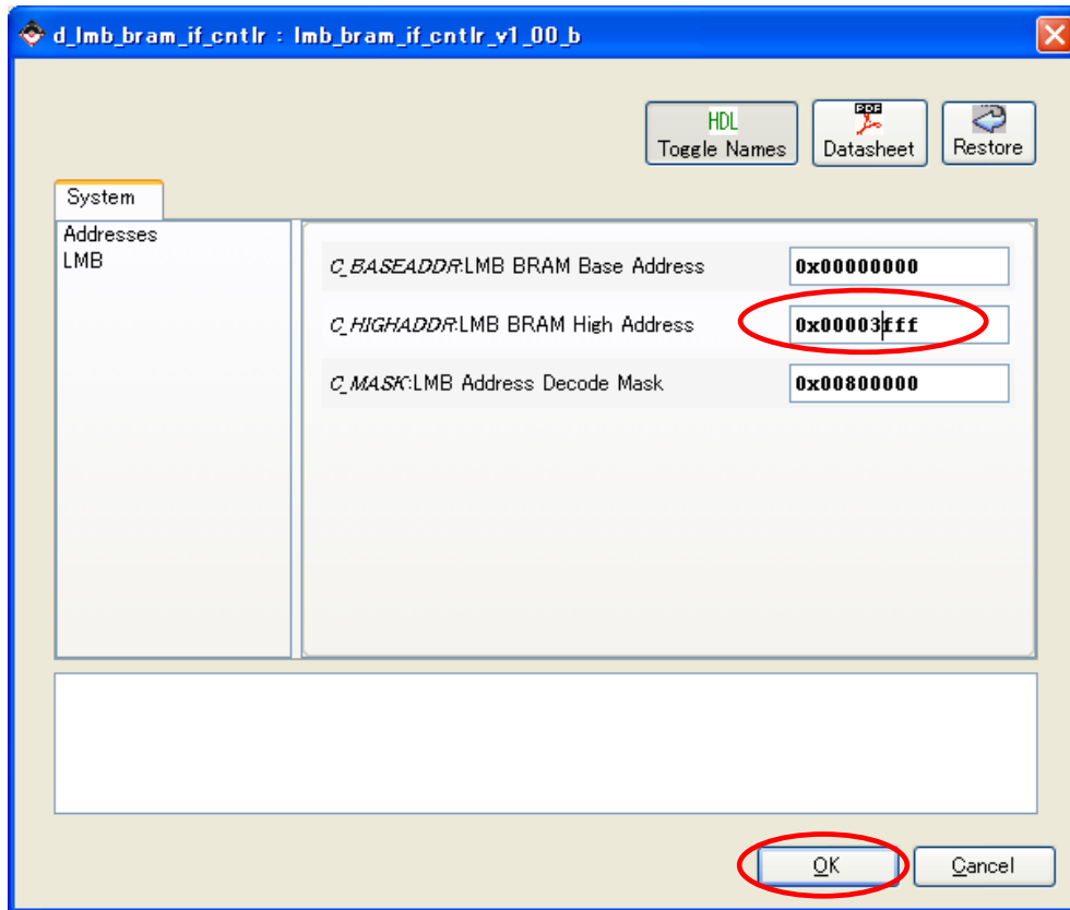
図 11-57 8kByte 16kByte に変更
