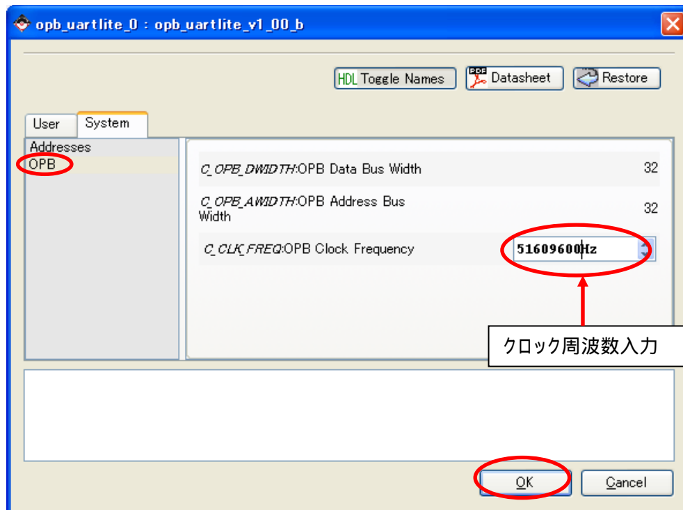
図 10-75 クロック周波数の設定
