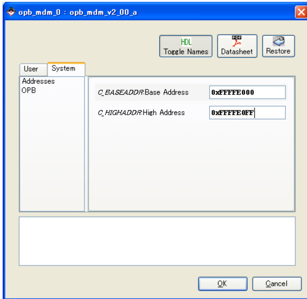
図 11-53 デバッガのアドレス設定
