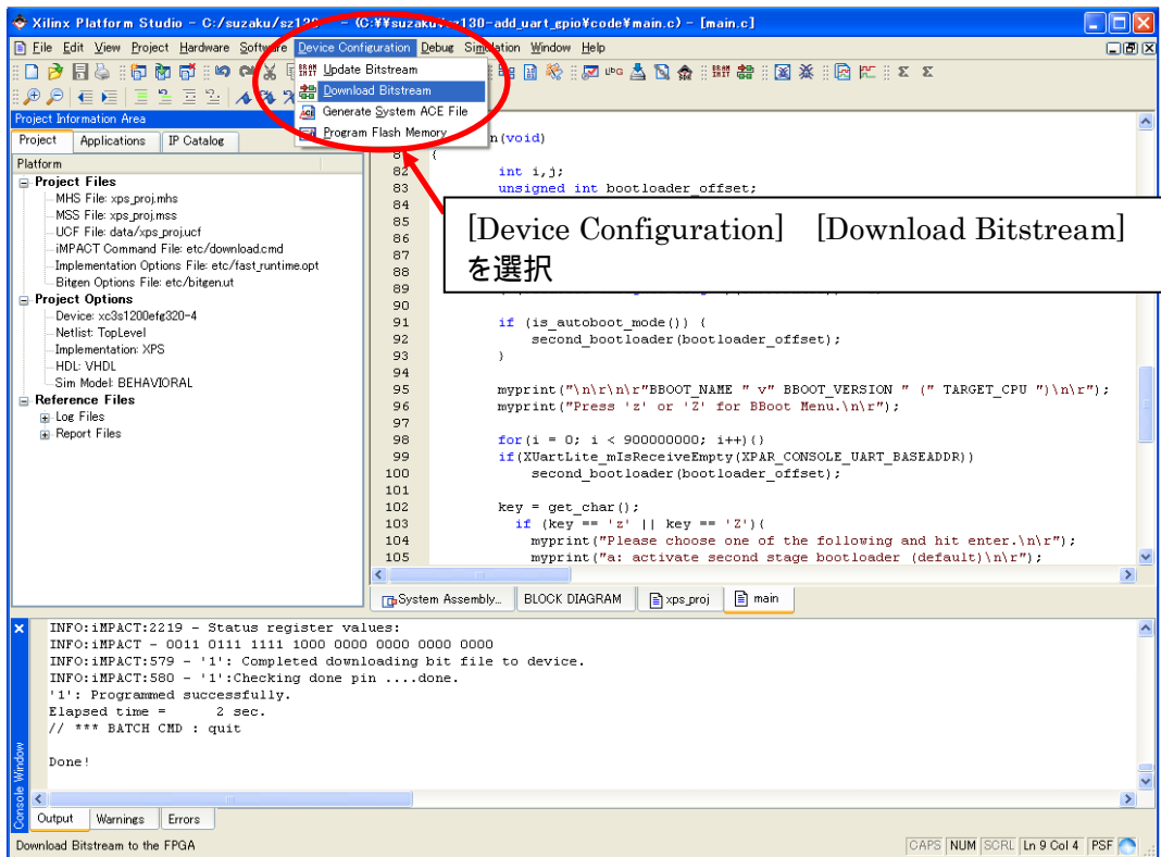
図 10-65 コンフィギュレーション
