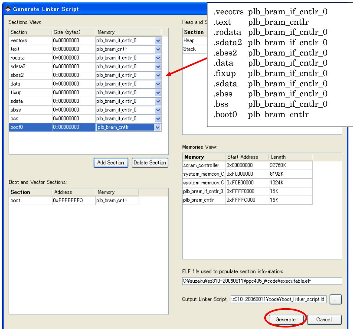
図 11-59 割り込み設定(リンカースクリプト設定: SZ310)
