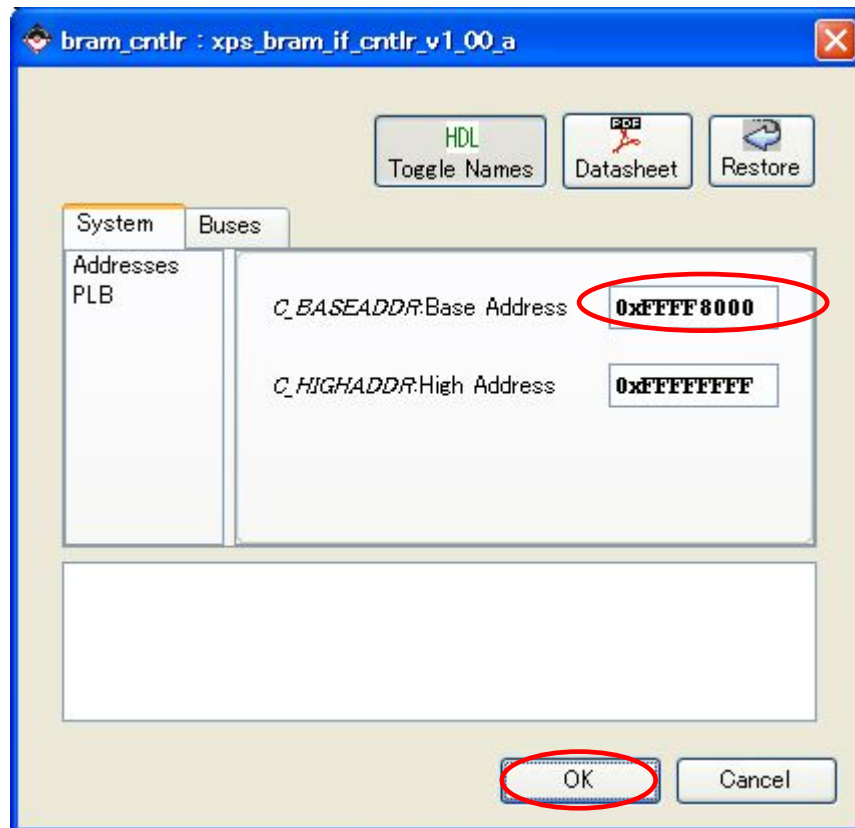
図 11-71 16KByte 32KByte に変更
