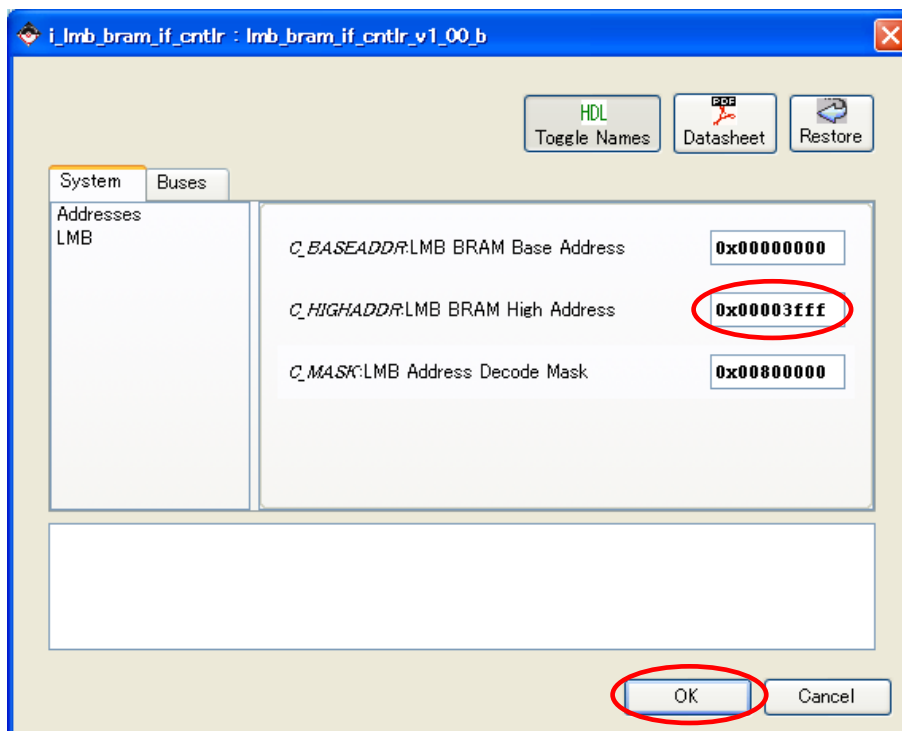
図 11-70 8KByte 16KByte に変更(i_lmb_bram_if_cntlr)
