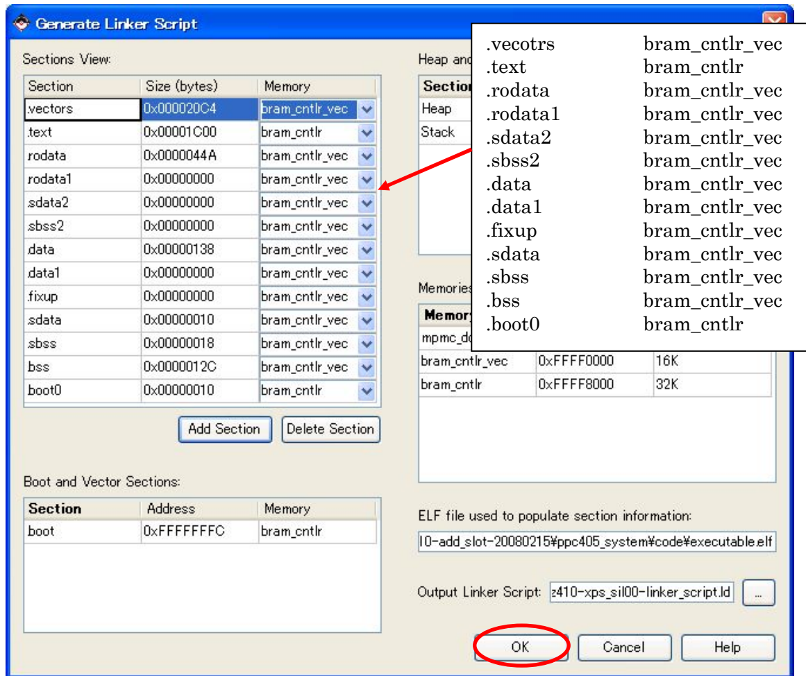
図 11-60 割り込み設定(リンカースクリプト設定: SZ410)
