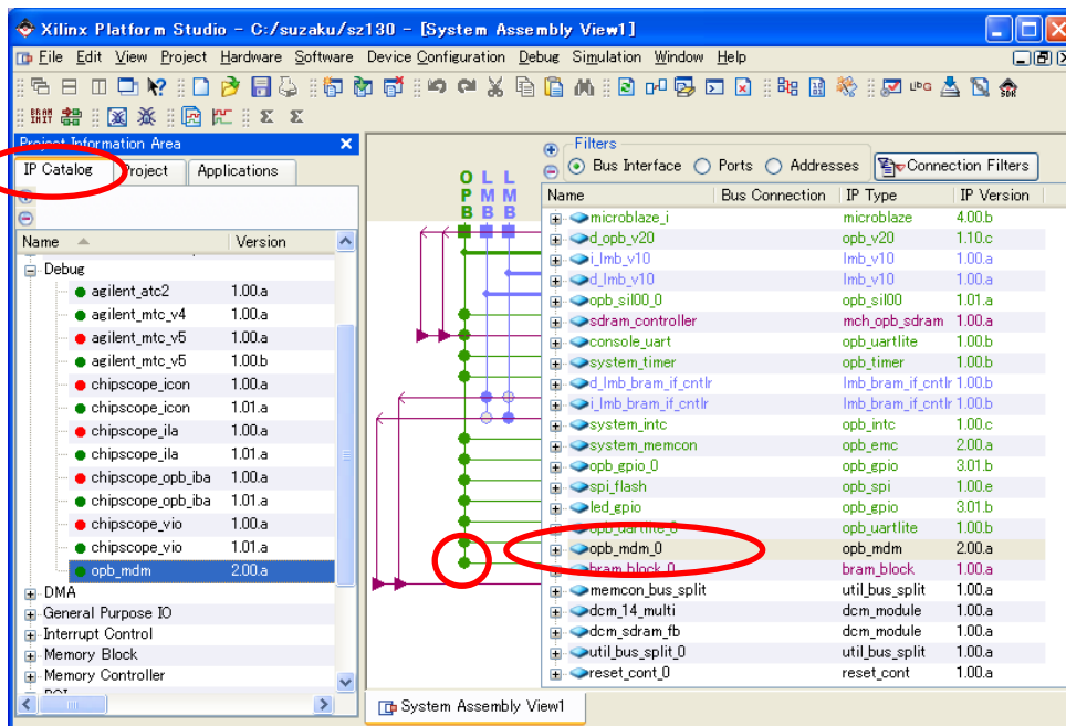
図 11-78 opb-mdm を追加してバスに接続
