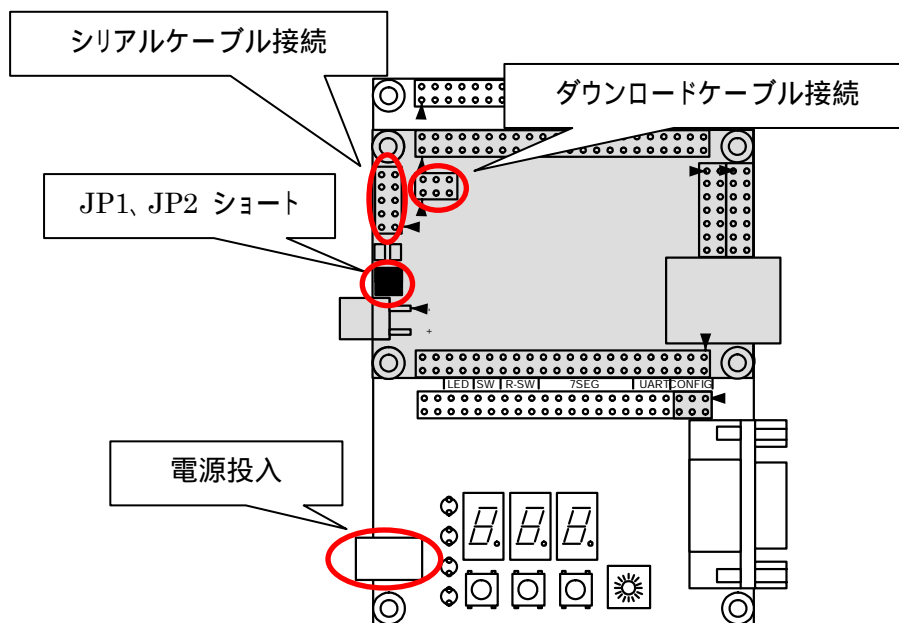
図 11-73 ジャンパの設定等
