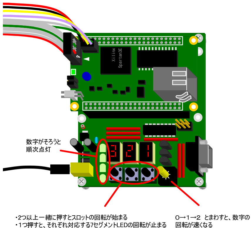
図 11-75 スロットマシン完成
