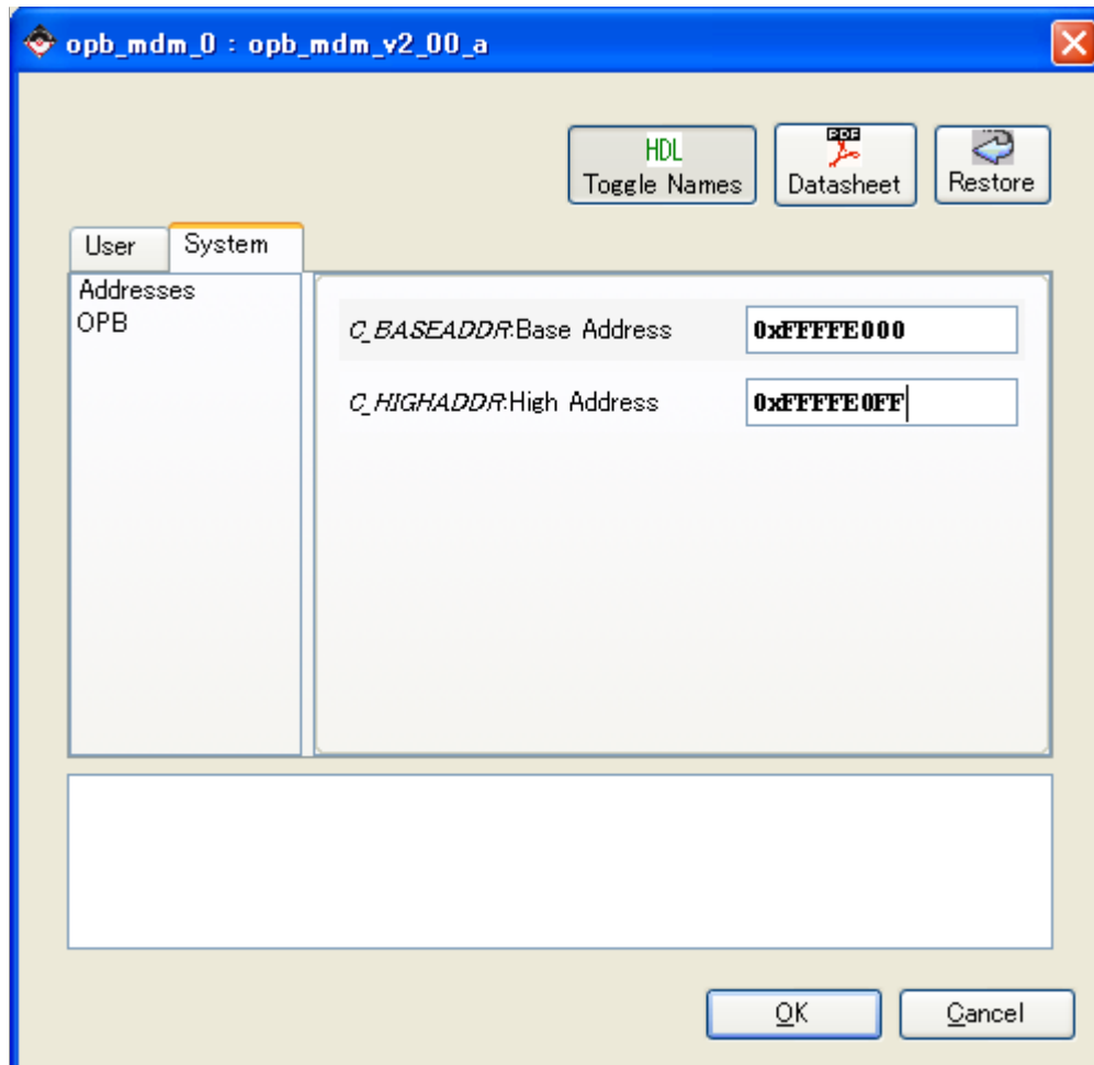
図 11-79 デバッガのアドレス設定
