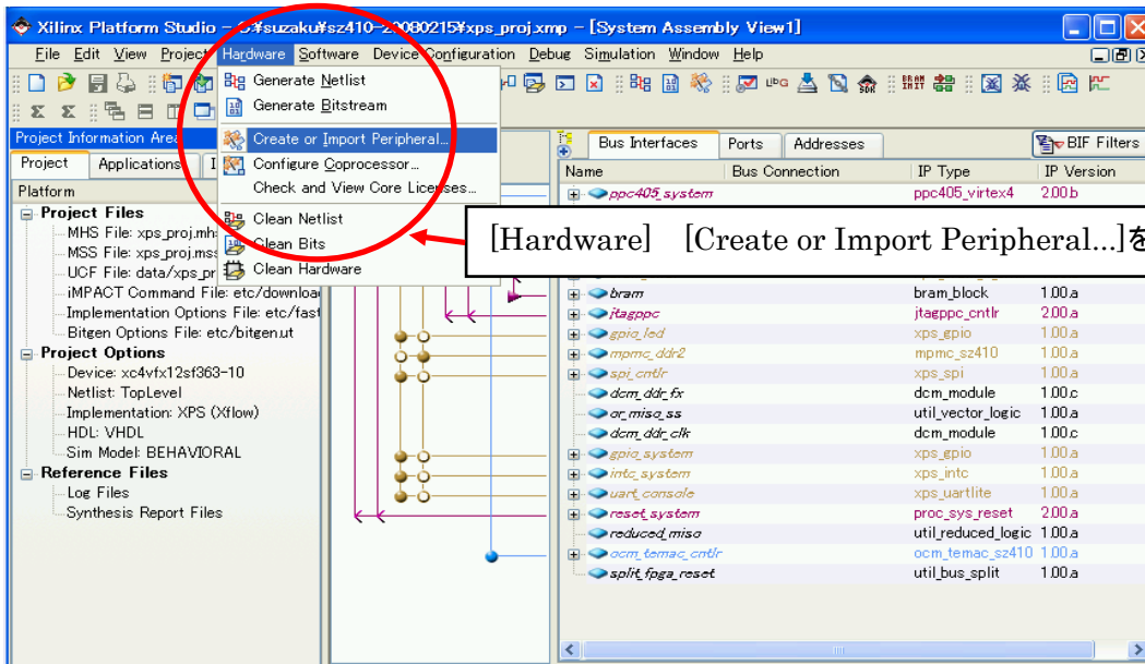
図 11-21 Create and Import Peripheral Wizard の起動のさせ方(EDK9.2i)
