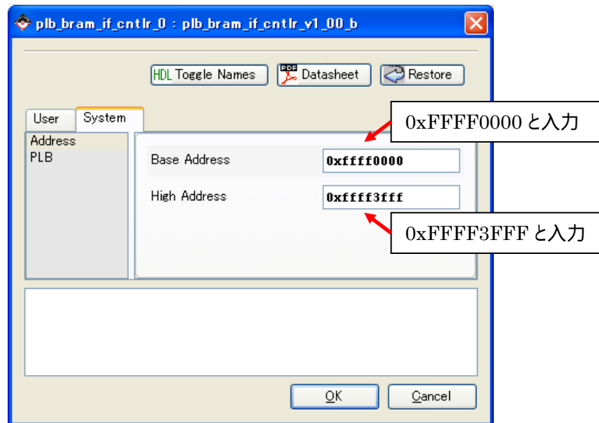
図 11-57 割り込み設定(アドレス変更)
