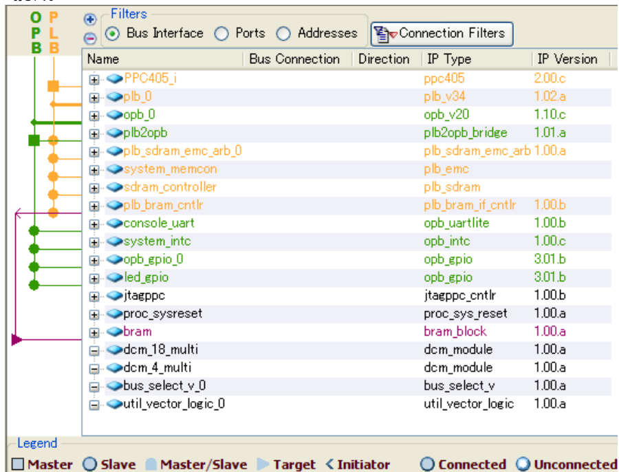
図 10-64 SZ310 のデフォルト(EDK)
