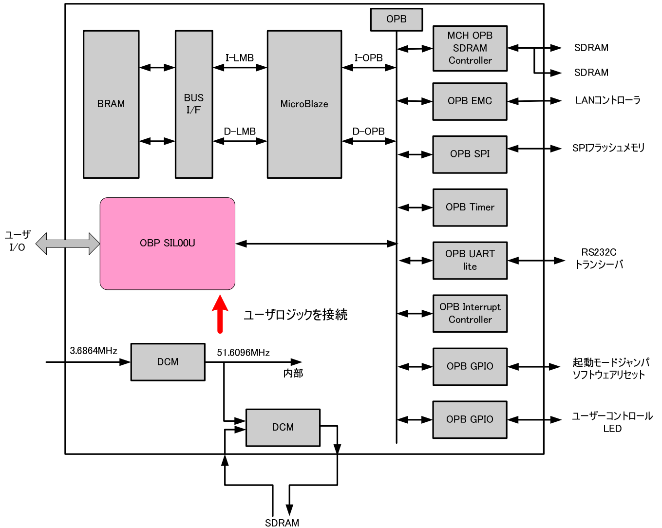
図 11-40 SZ130 のデフォルトに自作 IP コアを追加
