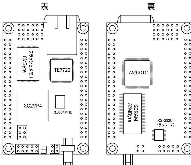
図 1-11 SUZAKU の主要部品配置図
