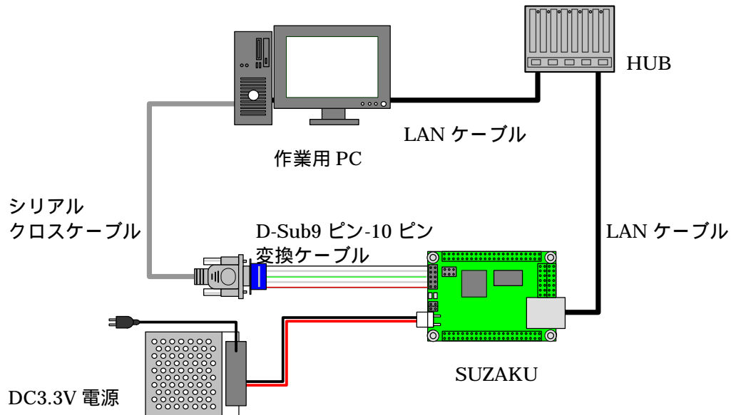
図 2-1 SUZAKU 接続例
