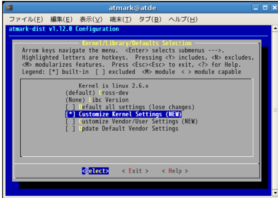
図 8.1. Customize Kernel Settings を選択
