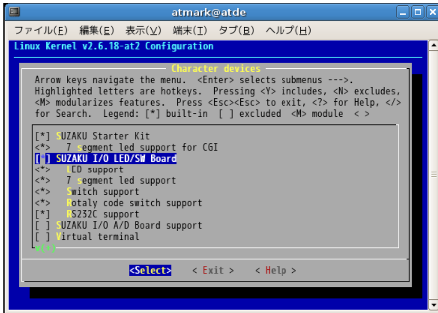
図 8.4. ドライバの追加
